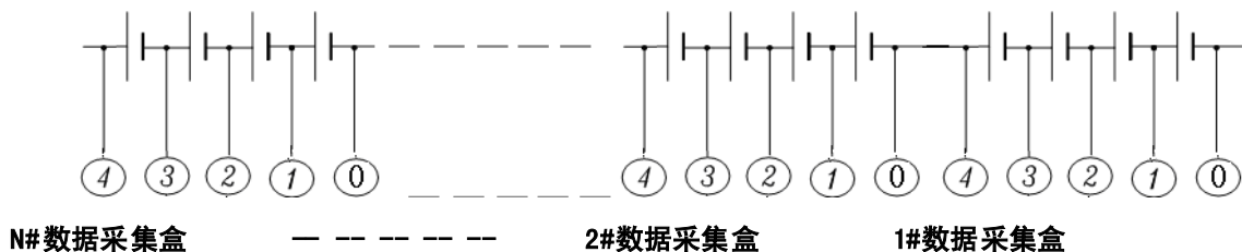
图 3.3 多个数据采集盒接线图
