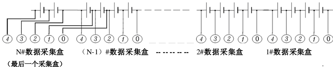
图 3.4 电池数量有多余时采集盒接线图
